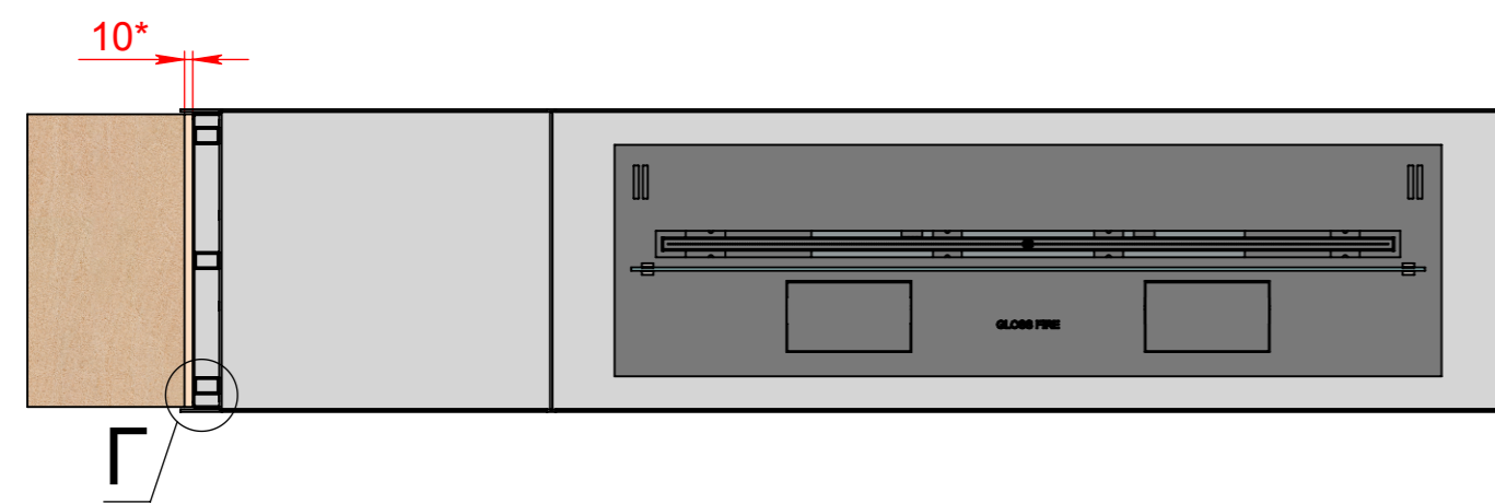
А-А (1 : 10)
