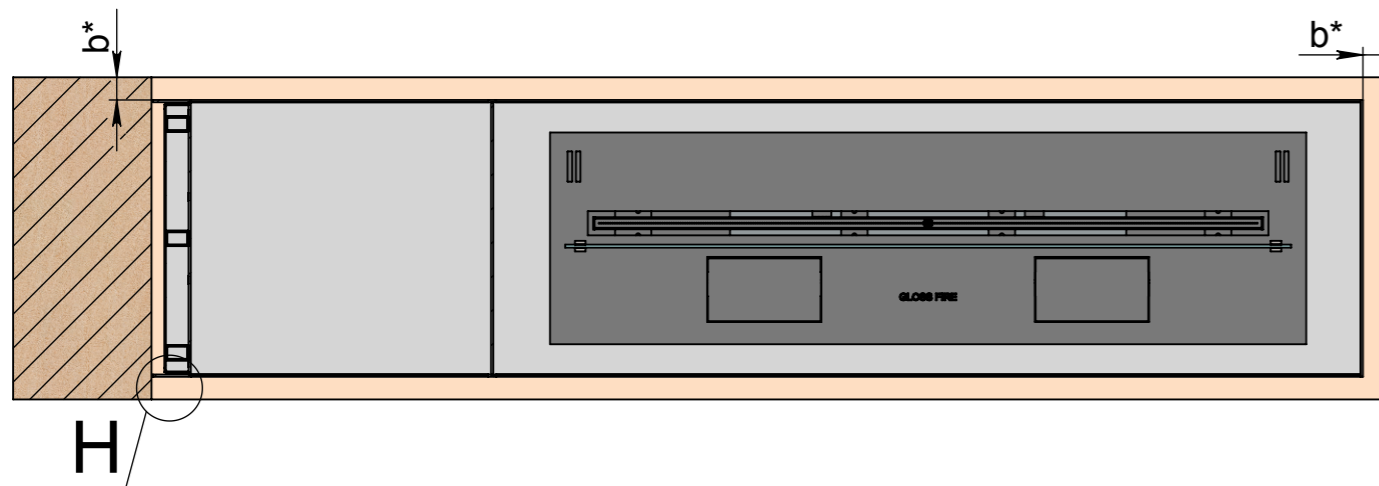
К-К (1 : 10)
