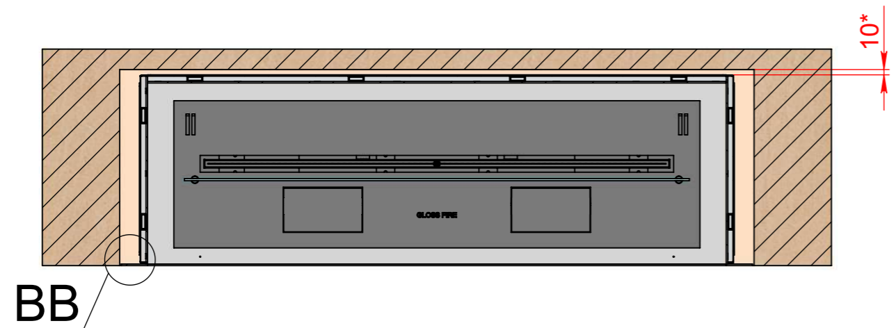
BA-BA (1 : 10)
