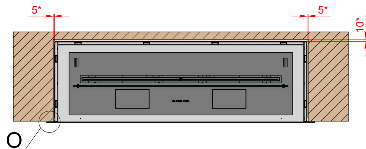
M-M (1 : 10)
