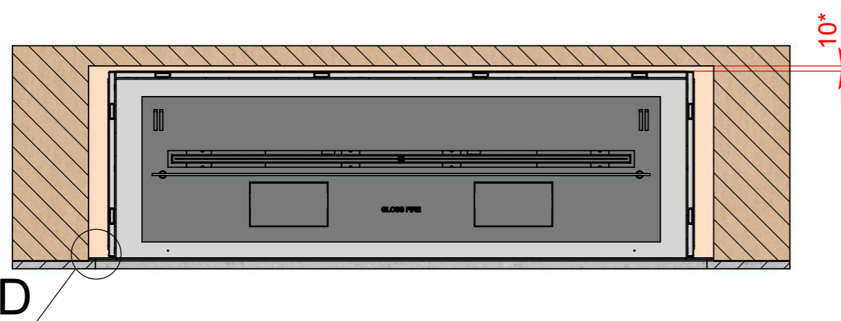
E-E (1 : 10)
