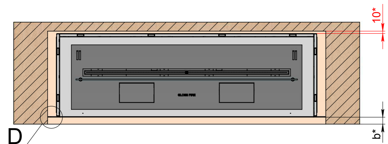
C-C (1 : 10)
