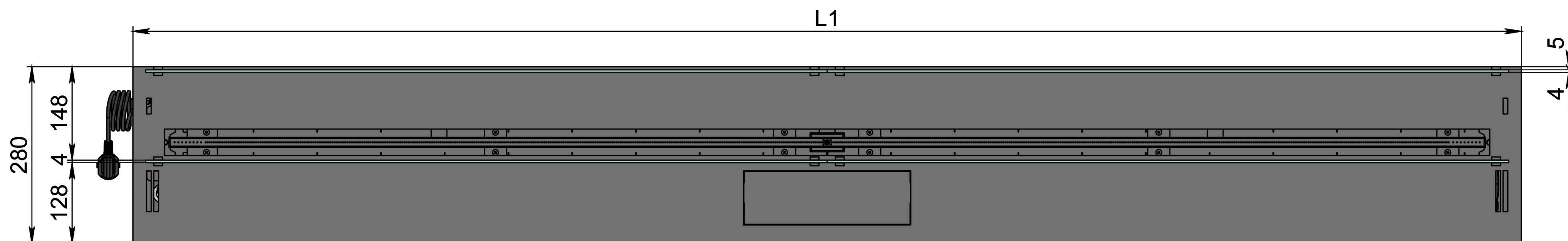
Вид сверху
