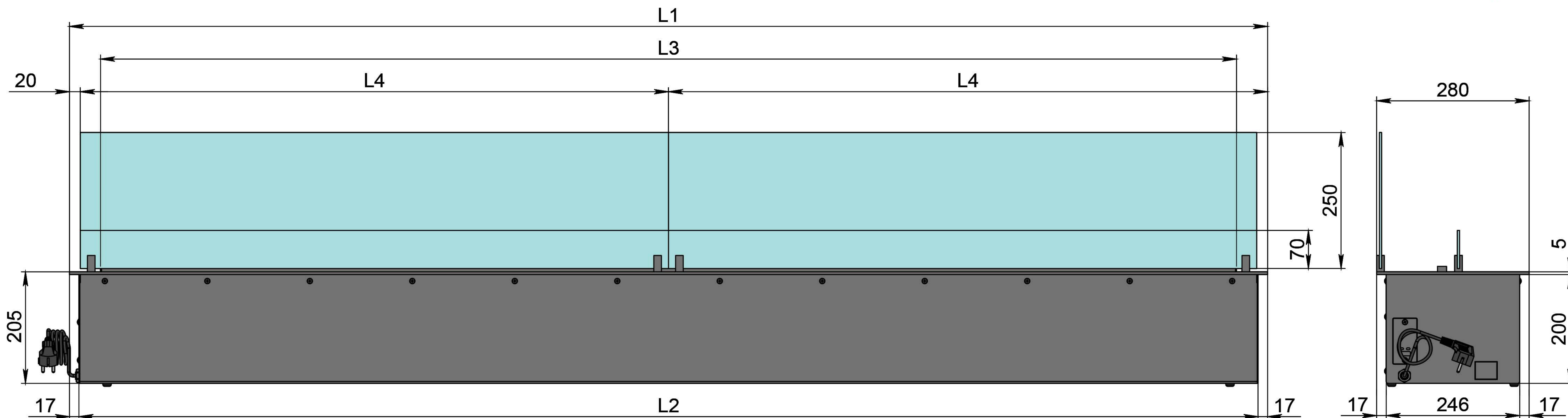
Вид сбоку
