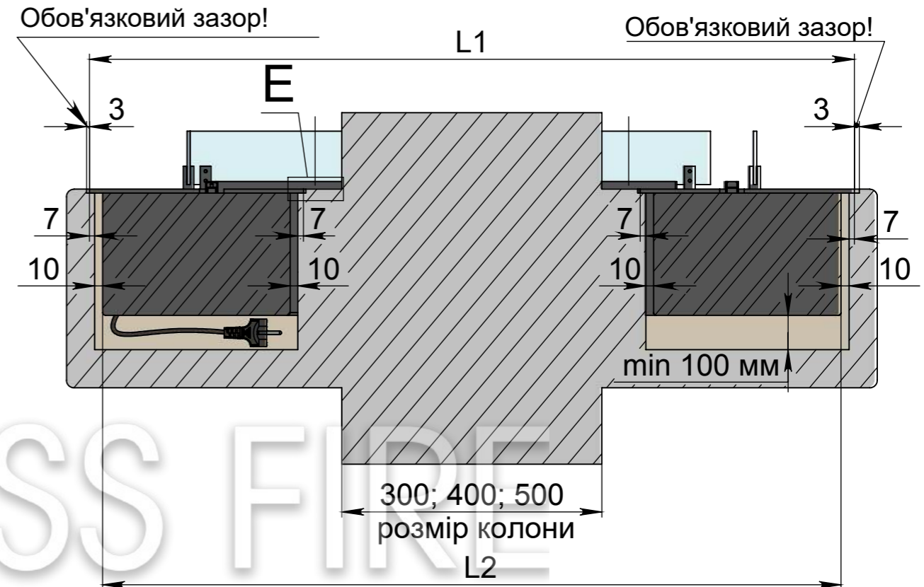
Розріз В-В
