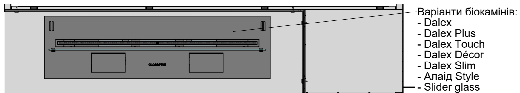
A-A (1 : 10)
