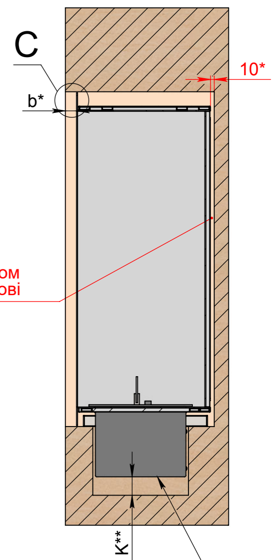
BC-BC (1 : 10)
